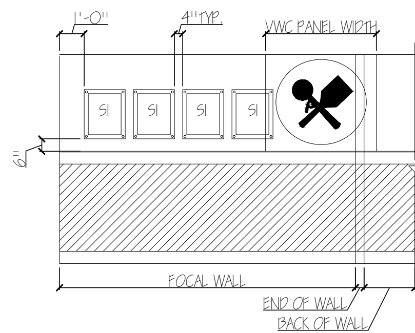
1 ELEV. - STORY WALL A-7 SCALE: 1/4" = 1'-0"
