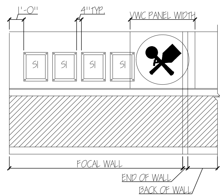
1 ELEV. - STORY WALL A-7 SCALE: 1/4" = 1'-0"
