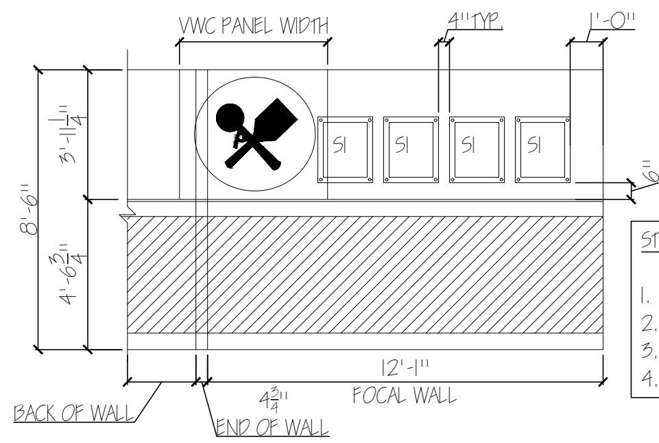
1 ELEV. - STORY WALL A-7 SCALE: 1/4" = 1'-0"
